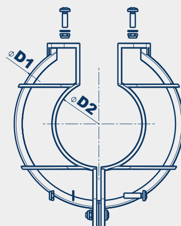
Dimensioni in mm
