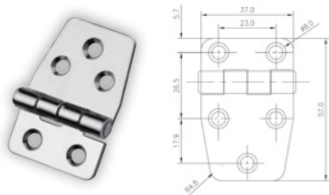
Bisagra, AISI 316, Dcha
