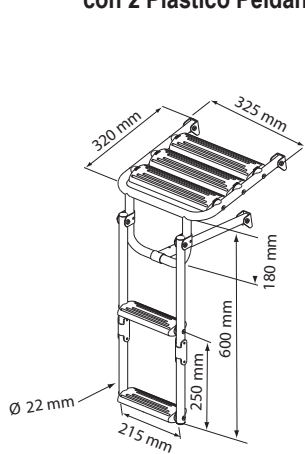
Plataforma Escalera, Inox 316, con 2 Plástico Peldaños
