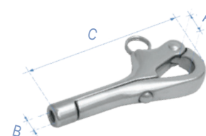
Gancho pelicano, Inox 316
