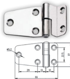
Bisagra Dcha con Angulo, Inox 316
