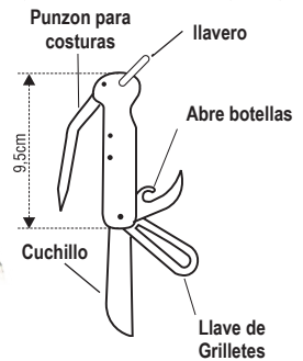
Cuchillo mariner "Skiper Mate", Acero Inoxidable, L:9,5 cm
