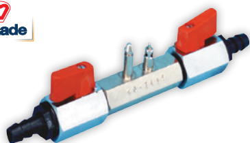
Valvula Combustible Doble Manguera Ø 10 mm
