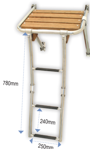
Plataforma Inox 316 con Escalera Plegable
