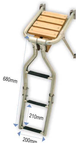
Plataforma Inox 316 con Escalera
