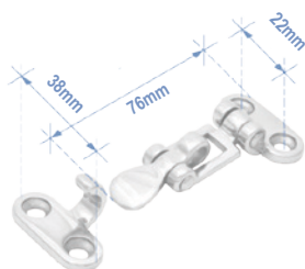
pestillo de la cubierta, Inox 316
