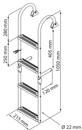
Escalera, Inox 316 plegable popa estrecha 2+2 Peldaños, 180°
