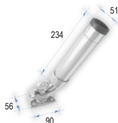
Cañero de cubierta, AISI 316
