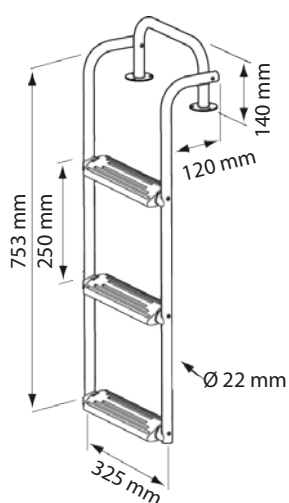
Escalera Plegable, Inoxidable 316, 3 Peldaños
