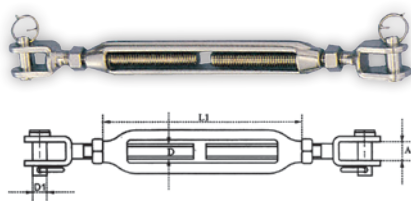
Tensor de marco con tuerca, mordaza y mordaza, Inox 316
