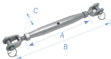
Tensor de tubería con tuerca, mordaza y mordaza, Inox 316
