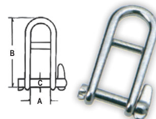
Grillete, Tipo Halyard, con Cross Bar & Pin Seguridad, Inox 316
