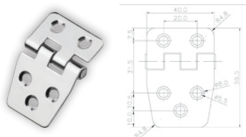
Bisagra, Invertida, Inox 316
