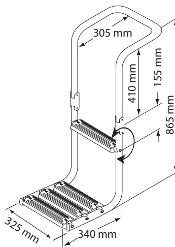
Plataforma Escalera submergida, Inox 316
