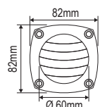
Tapa tubería de ventilación, PA
