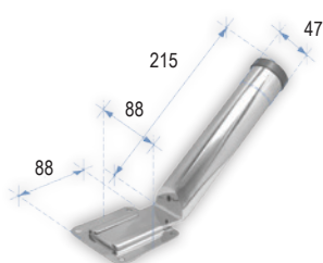
Cañero, Desmontable, Inox 304
