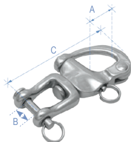
Grillete a presión, con mordaza giratoria de fundición, AISI 316
