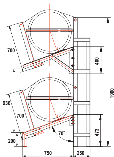
Soporte vertical para SOLAS OCEANO, 2-altos, 6-25(A), 6-35(B)
