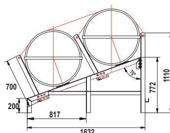
Soporte doble SOLAS OCEANO, 30-35(A)
