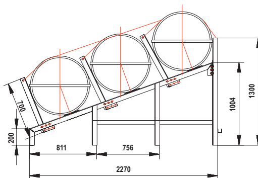
Soporte SOLAS OCEANO, triple, 6-25(A), 6-35(B)
