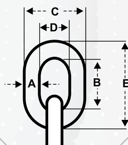
Dimensiones (mm)
